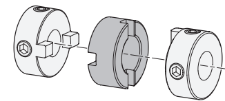
Montážní pokyny
